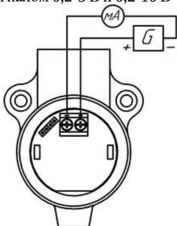
Рисунок 23в – преобразователь в корпусе И с выходным сигналом 4-20 мА
