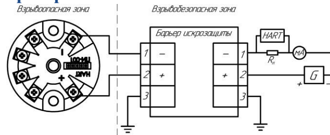
Рисунок 34в – подключение преобразователя с взрывозащитой Exia «искробезопасная электрическая цепь» в корпусе К с выходным сигналом 4-20 мА – HART
