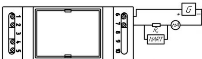
Рисунок 25в – преобразователь в корпусе Д с выходным сигналом 4-20 мА – HART
