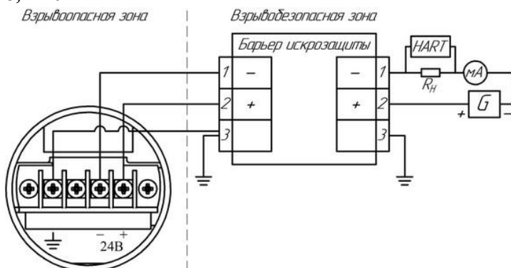
Рисунок 42в – подключение преобразователя с взрывозащитой Exia «искробезопасная электрическая цепь» в корпусе Т, Ти с выходным сигналом 4-20 мА – HART
