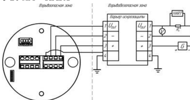
Рисунок 41в – подключение преобразователя с взрывозащитой Exia «искробезопасная электрическая цепь» в корпусе П, Пи с выходным сигналом 0,2-5 В и 0,2-10 В – HART
