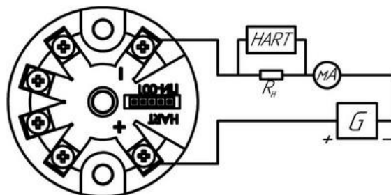
Рисунок 19в – преобразователь в корпусе К с выходным сигналом 4-20 мА – HART
