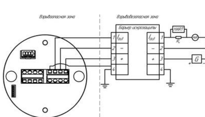
Рисунок 40в – подключение преобразователя с взрывозащитой Exia «искробезопасная электрическая цепь» в корпусе П, Пи с выходным сигналом 0-5 мА и 0-20 мА – HART
