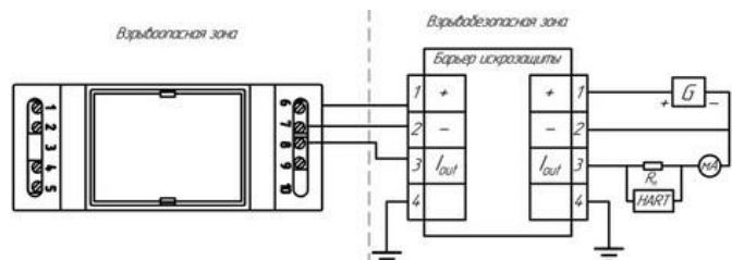
Рисунок 37в – подключение преобразователя с взрывозащитой Exia «искробезопасная электрическая цепь» в корпусе Д с выходным сигналом 0-5 мА и 0-20 мА – HART
