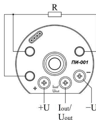
Рисунок 10в – преобразователь в корпусе Е, выходной сигнал 0-5 мА, 0-20 мА, 0,2-5 В и 0,2-10 В
