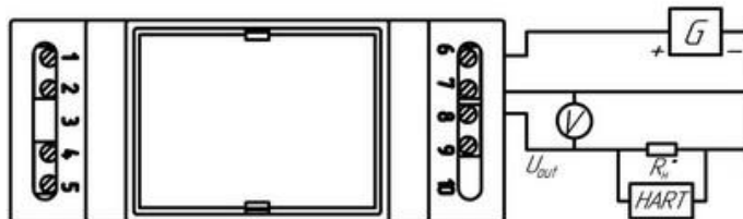
Рисунок 27в – преобразователь в корпусе Д с выходным сигналом 0,2-5 В и 0,2-10 В – HART
