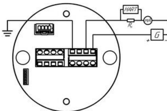
Рисунок 28в – преобразователь в корпусе П, Пи с выходным сигналом 4-20 мА – HART
