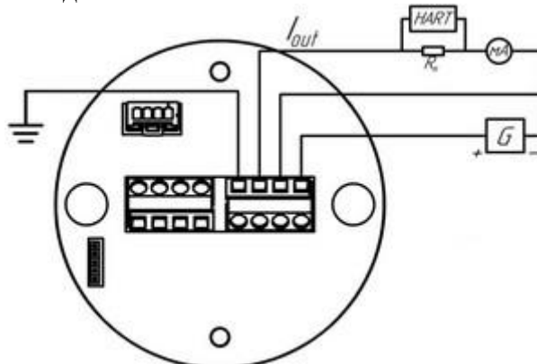
Рисунок 29в – преобразователь в корпусе П, Пи с выходным сигналом 0-5 мА и 0-20 мА – HART
