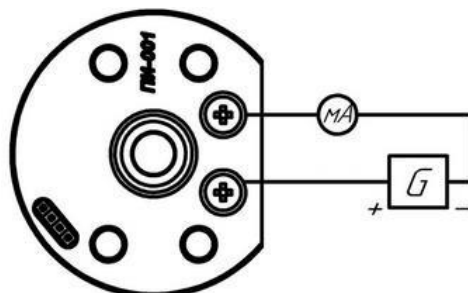
Рисунок 20в – преобразователь в корпусе Е с выходным сигналом 4-20 мА
