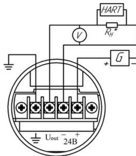
Рисунок 33в – преобразователь в корпусе Т, Ти с выходным сигналом 0,2-5 В и 0,2-10 В – HART
