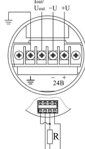
Рисунок 16в – преобразователь в корпусе Т, Ти, выходной сигнал 0-5 мА, 0-20 мА, 0,2-5 В и 0,2-10 В
