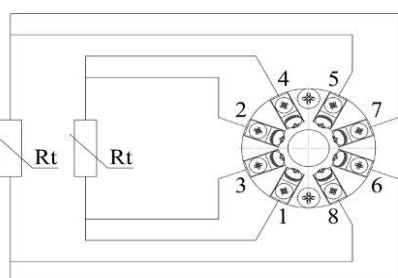
Рисунок 6в - ТС с двумя элементами и четырехпроводной схемой подключения (2х4)
