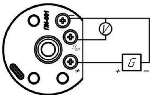
Рисунок 22в – преобразователь в корпусе Е с выходным сигналом 0,2-5 В и 0,2-10 В
