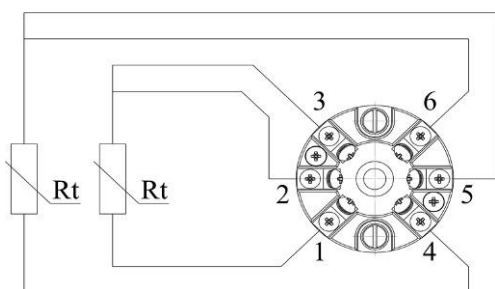
Рисунок 5в - ТС с двумя элементами и трехпроводной схемой подключения (2х3)
