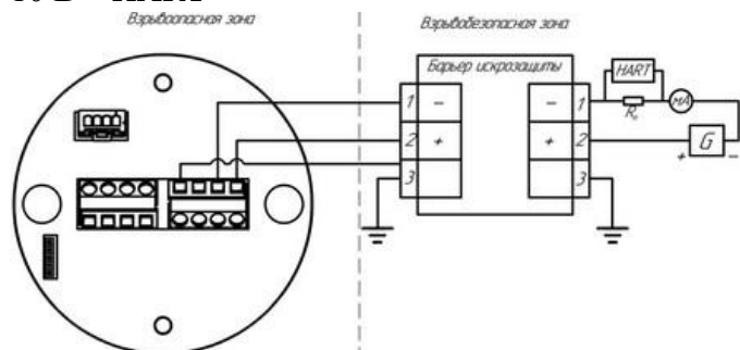
Рисунок 39в – подключение преобразователя с взрывозащитой Exia «искробезопасная электрическая цепь» в корпусе П, Пи с выходным сигналом 4-20 мА – HART
