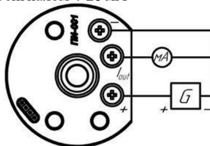
Рисунок 20в – преобразователь в корпусе Е с выходным сигналом 4-20 мА
