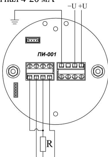
Рисунок 13в – преобразователь в корпусе П, Пи, выходной сигнал 4-20 мА – HART
