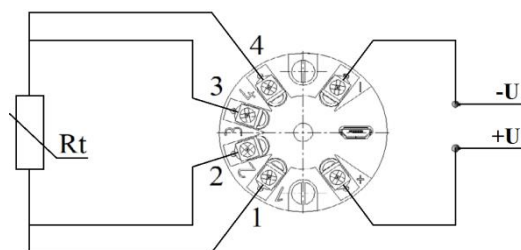
Рисунок 7в - ТС-Б-У с четырехпроводной схемой подключения (х4)
