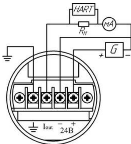
Рисунок 32в – преобразователь в корпусе Т, Ти с выходным сигналом 0-5 мА и 0-20 мА – HART
