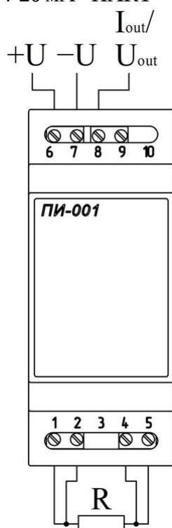
Рисунок 18в – преобразователь в корпусе Д, выходной сигнал 0-5 мА, 0-20 мА, 0,2-5 В и 0,2-10 В
