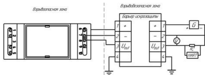
Рисунок 38в – подключение преобразователя с взрывозащитой Exia «искробезопасная электрическая цепь» в корпусе Д с выходным сигналом 0,2-5 В и 0,2-10 В – HART
