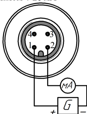
Рисунок 24в – преобразователь в трубном корпусе 4Р с выходным сигналом 4-20 мА
