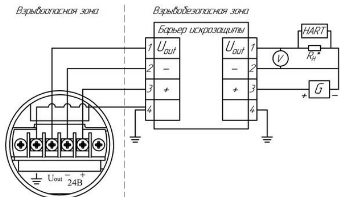
► Рисунок 44в – подключение преобразователя с взрывозащитой Exia «искробезопасная электрическая цепь» в корпусе Т, Ти с выходным сигналом 0,2-5 В и 0,2-10 В – HART
