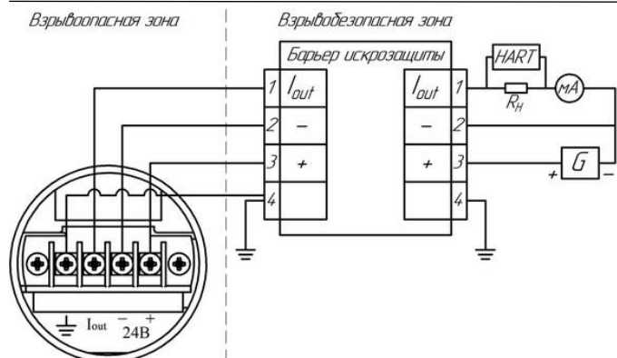
► Рисунок 43в – подключение преобразователя с взрывозащитой Exia «искробезопасная электрическая цепь» в корпусе Т, Ти с выходным сигналом 0-5 мА и 0-20 мА – HART
