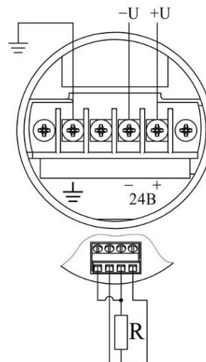
Рисунок 15в – преобразователь в корпусе Т, Ти, выходной сигнал 4-20 мА - HART
