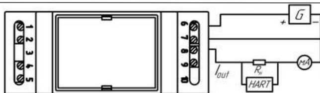
Рисунок 26в – преобразователь в корпусе Д с выходным сигналом 0-5 мА и 0-20 мА – HART
