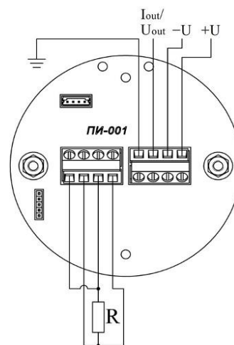
Рисунок 14в – преобразователь в корпусе П, Пи, выходной сигнал 0-5 мА, 0-20 мА, 0,2-5 В и 0,2-10 В
