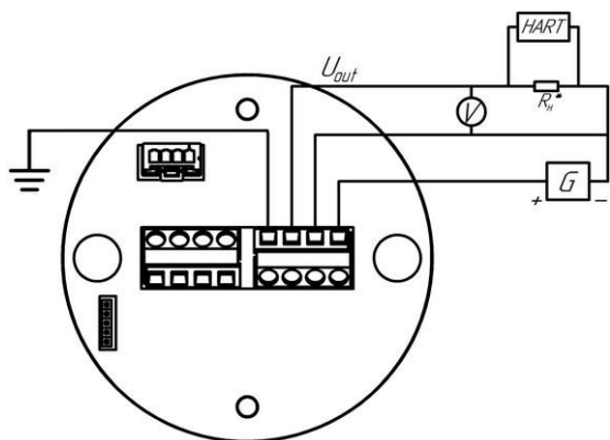
Рисунок 30в – преобразователь в корпусе П, Пи с выходным сигналом 0,2-5 В и 0,2-10 В – HART
