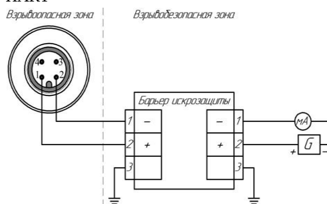
Рисунок 35в – подключение преобразователя с взрывозащитой Exia «искробезопасная электрическая цепь» в трубном корпусе К с выходным сигналом 4-20 мА
