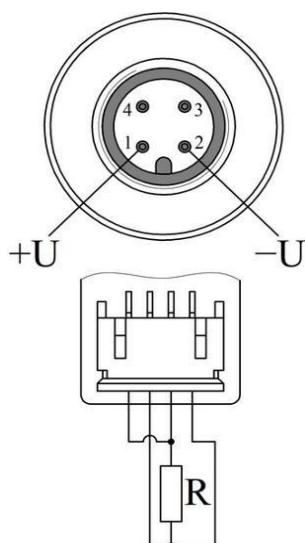
Рисунок 11в – преобразователь в трубном корпусе 4Р, выходной сигнал 4-20 мА
