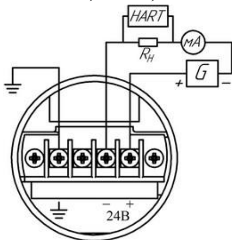
Рисунок 31в – преобразователь в корпусе Т, Ти с выходным сигналом 4-20 мА – HART
