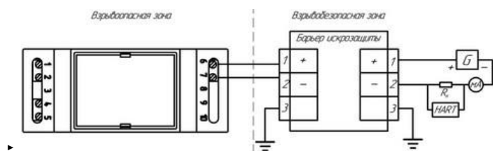
Рисунок 36в – подключение преобразователя с взрывозащитой Exia «искробезопасная электрическая цепь» в корпусе Д с выходным сигналом 4-20 мА – HART
